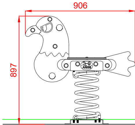
ALZADO
