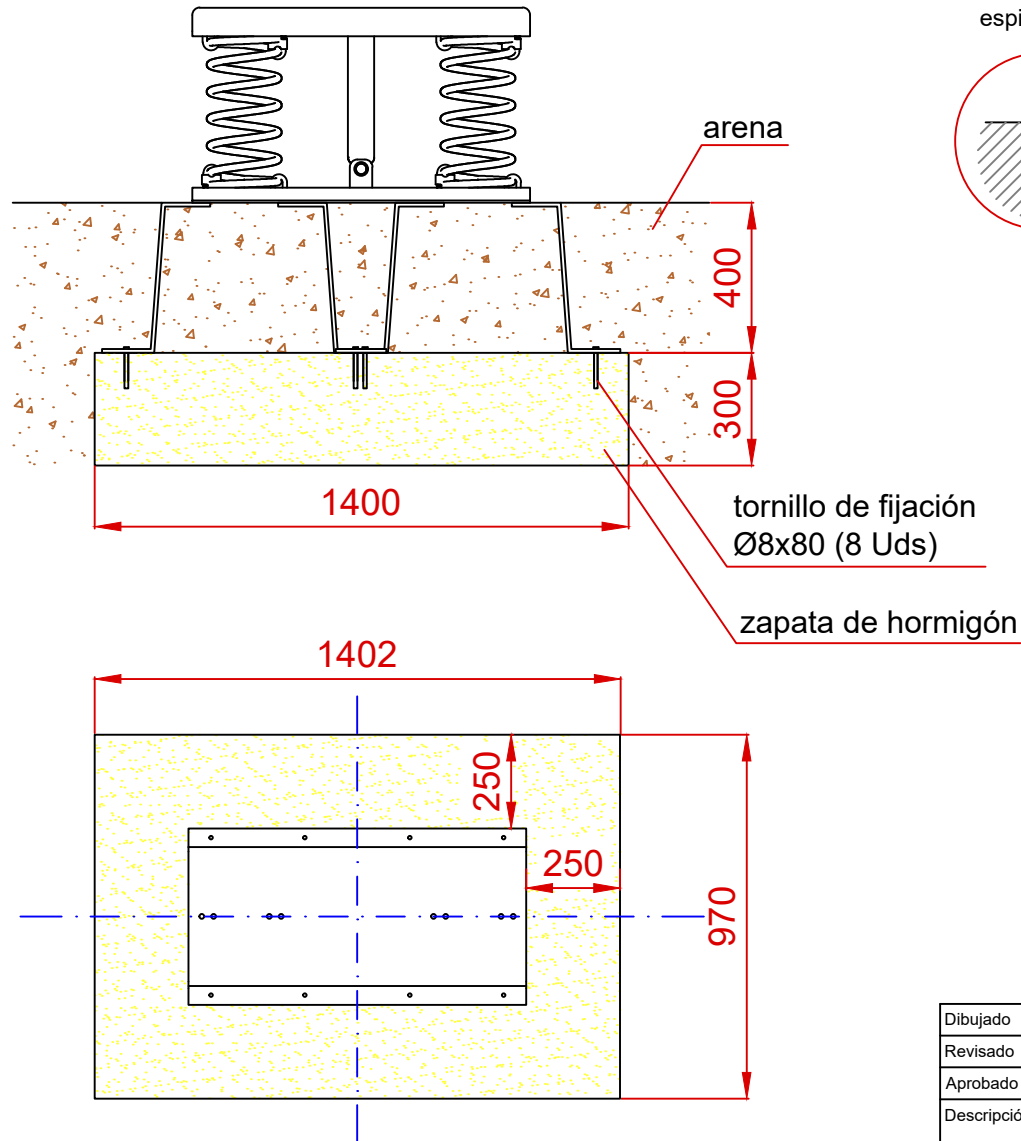
ESQUEMA DE CIMENTACIÓN EN ARENA
