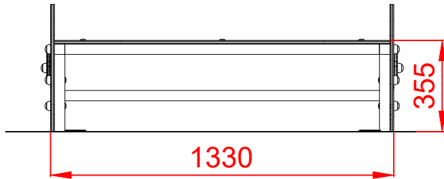
ALZADO
