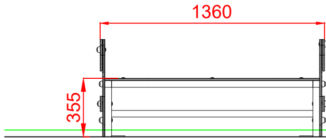
ALZADO
