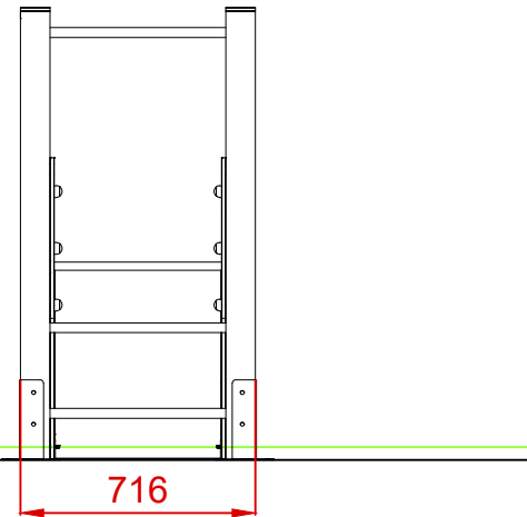
PERFIL IZQUIERDO
