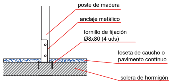
ESQUEMA DE CIMENTACIÓN EN HORMIGÓN E: 2/1
