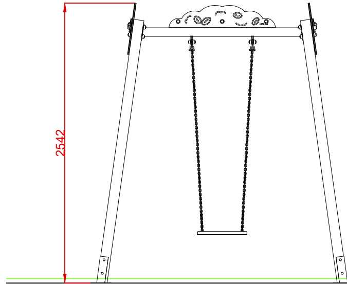
ALZADO
