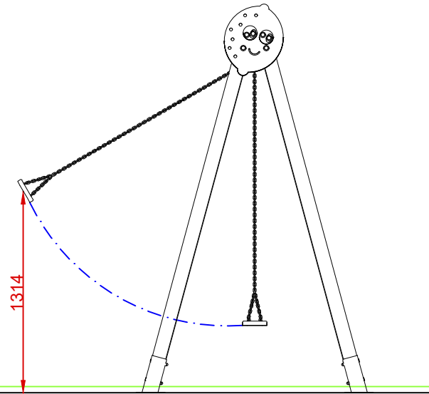
PERFIL
