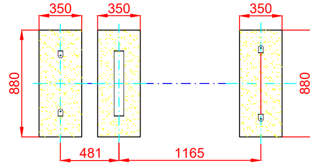
PLANTA CIMENTACIÓN
