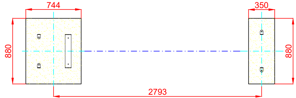
PLANTA CIMENTACIÓN
