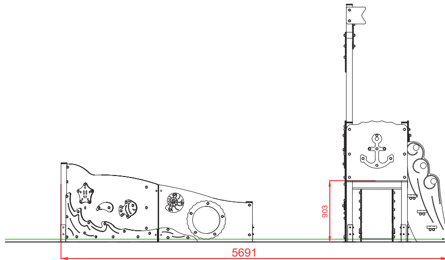
ALZADO
