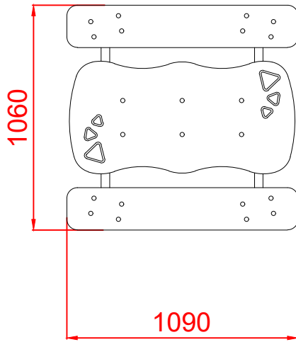
PLANTA
