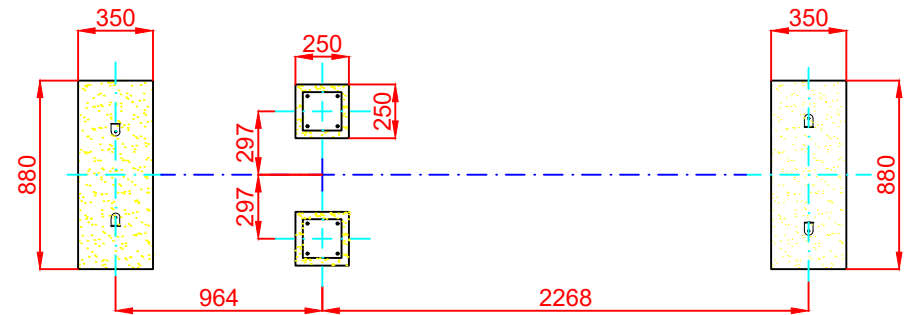
PLANTA CIMENTACIÓN
