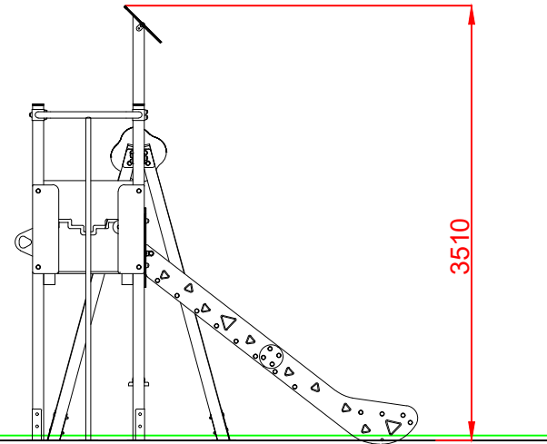
PERFIL IZQUIERDO
