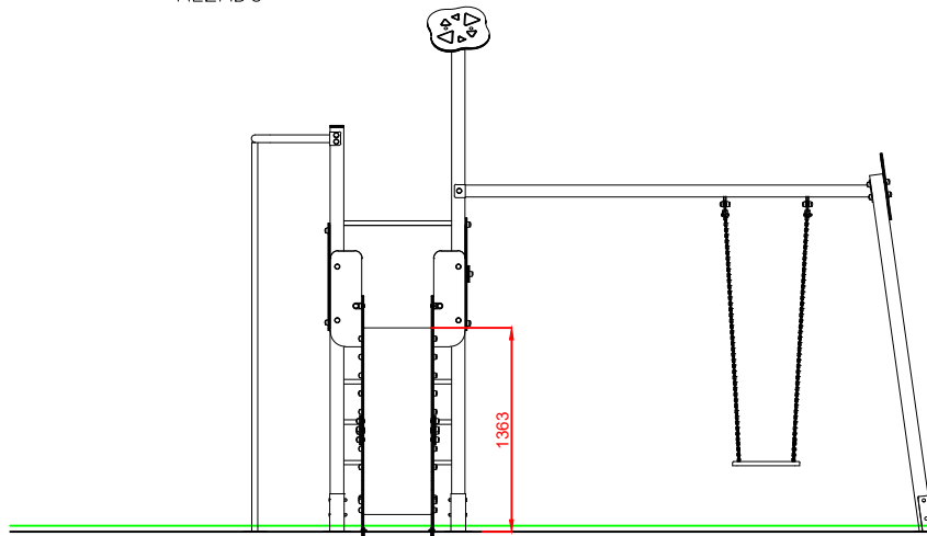
ALZADO
