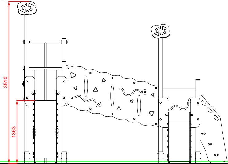
ALZADO
