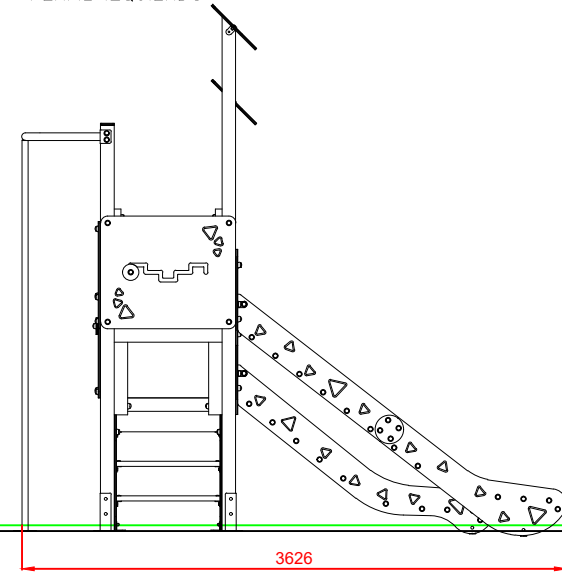
PERFIL IZQUIERDO
