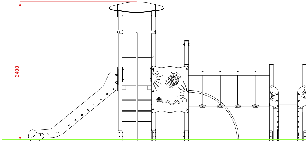
ALZADO
