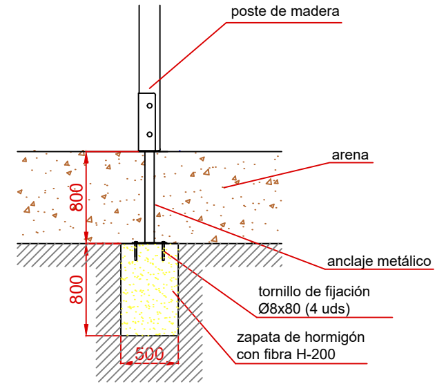
ESQUEMA DE CIMENTACIÓN EN ARENA E: 2/1
