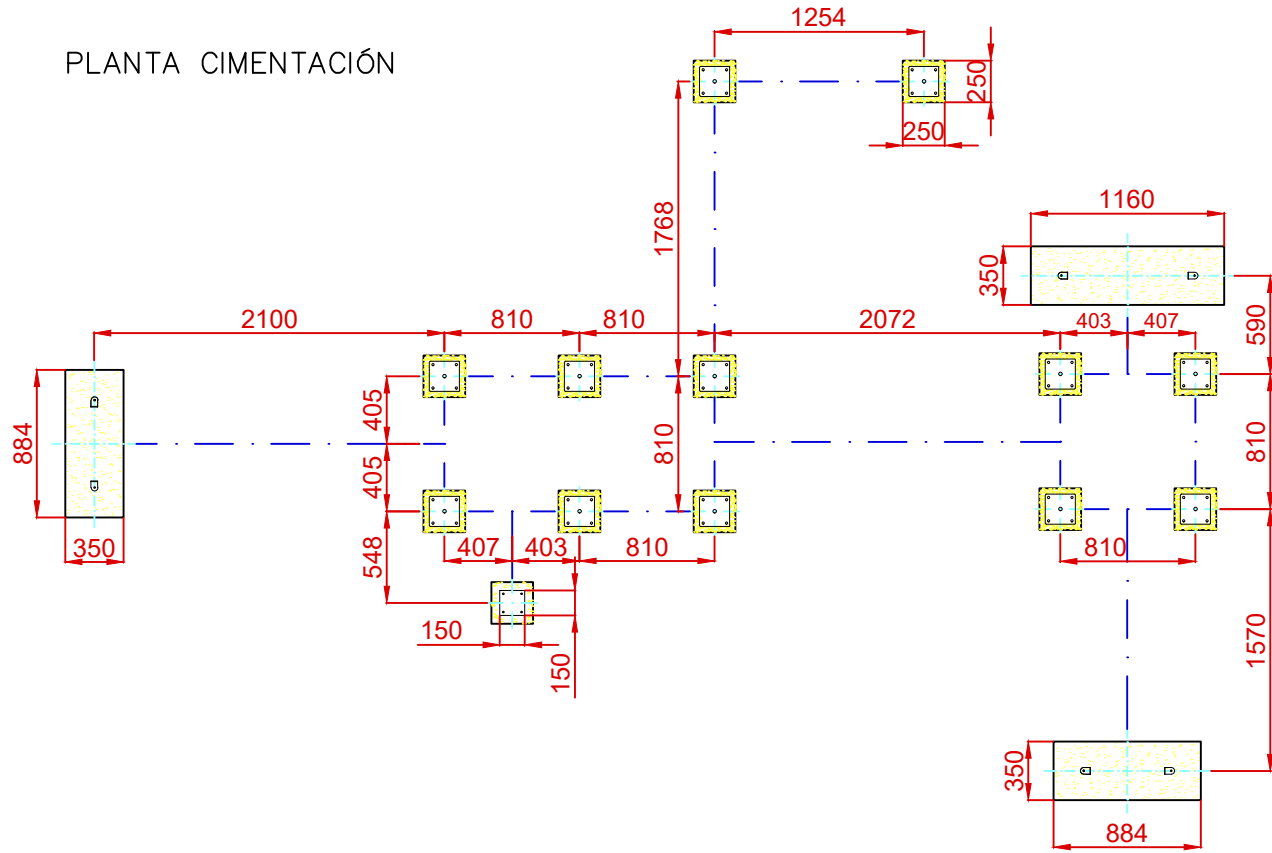
ESQUEMA DE CIMENTACIÓN EN HORMIGÓN E: 2/1
