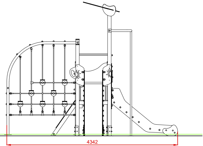
PERFIL
