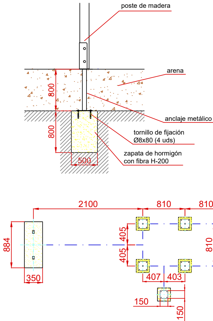
ESQUEMA DE CIMENTACIÓN EN ARENA E: 2/1
