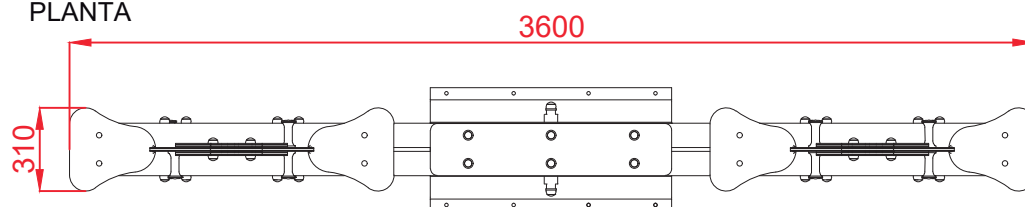
PLANTA
