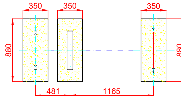
PLANTA CIMENTACIÓN
