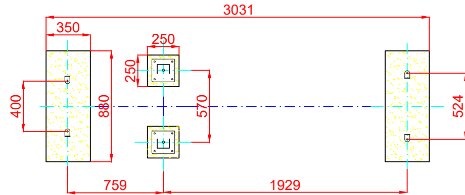
PLANTA CIMENTACIÓN
