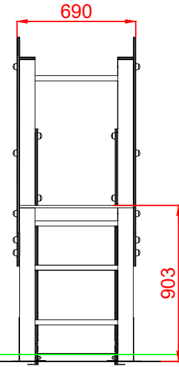
PERFIL
