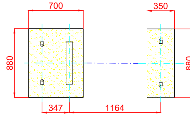
PLANTA CIMENTACIÓN
