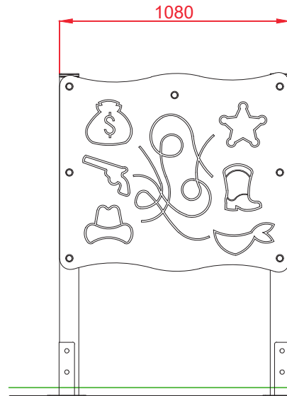
ALZADO
